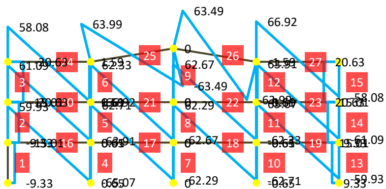
Ca.Tel.2D - Taglio [kN]
